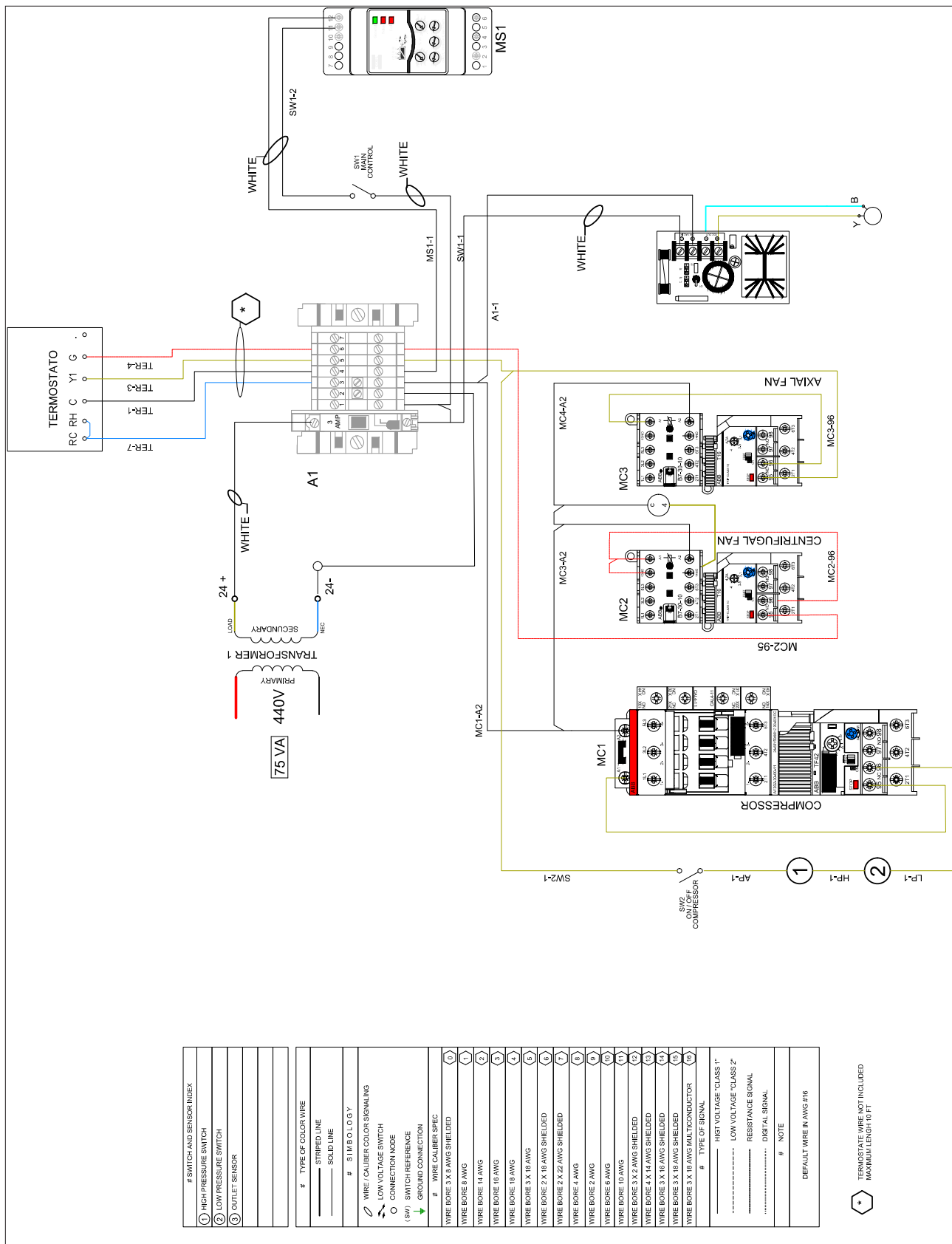
Figura 8. Diagrama solo frío 5TR 440V
